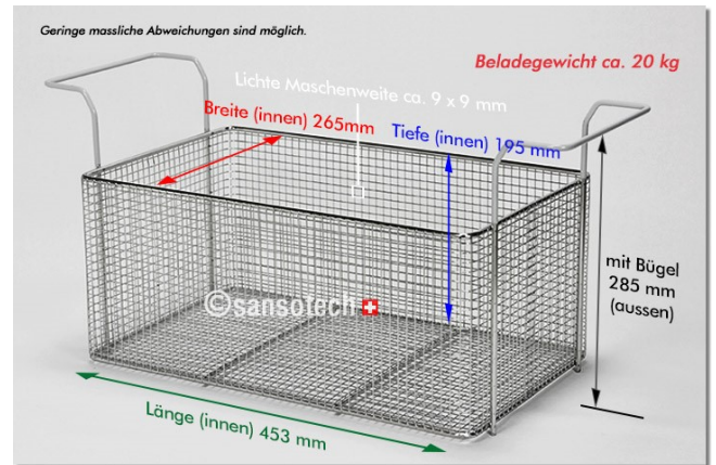
Wannenkorb (Edelstahl), neu Artikel-Nr. KBSW45H
